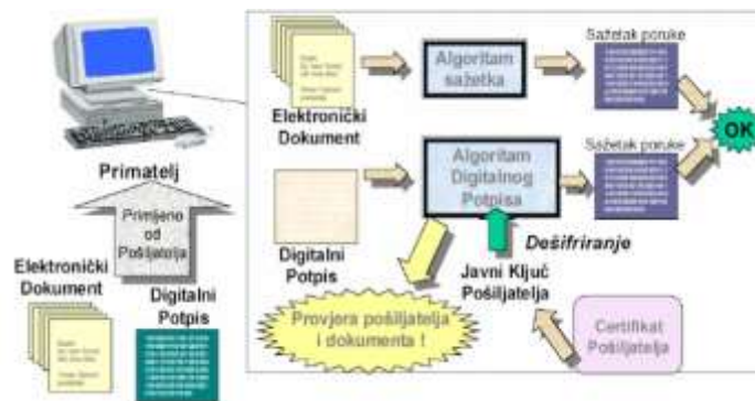
Slika 6. Digitalni Potpis - Provera
